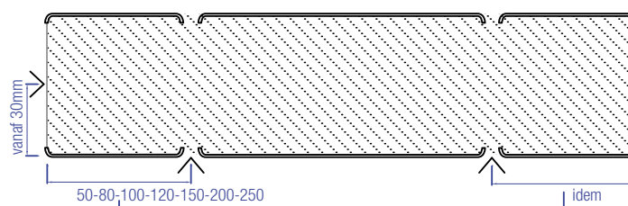
Type 4 Wand met 2 zaagsnedes
