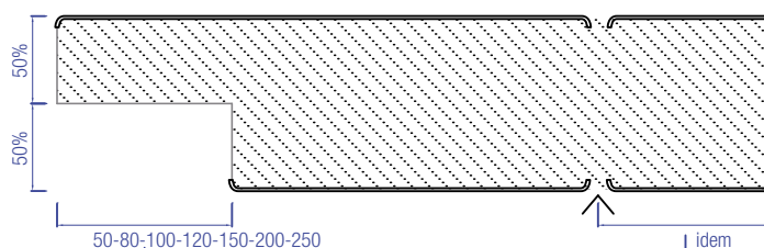
Type 2 Wand met inkeping en extra zaagsnede (beide zijden dezelfde kleur, niet met micro-profilering)
