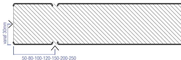
Type 3 Wand met zaagsnede
