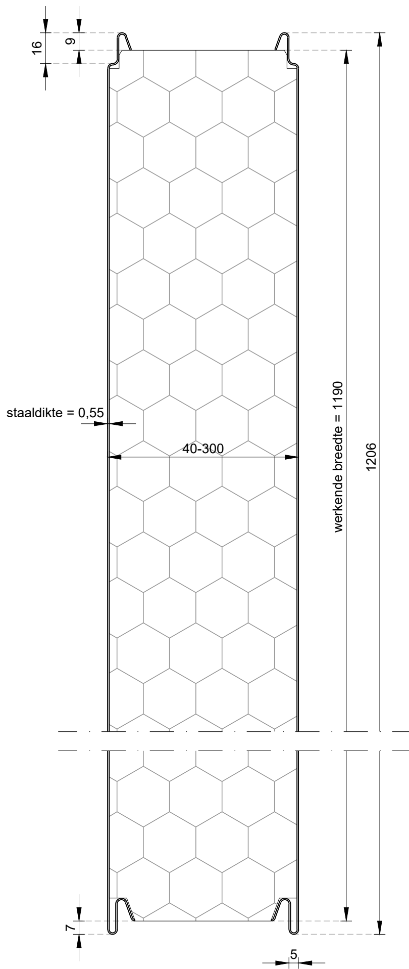
Doorsnede EPS paneel
