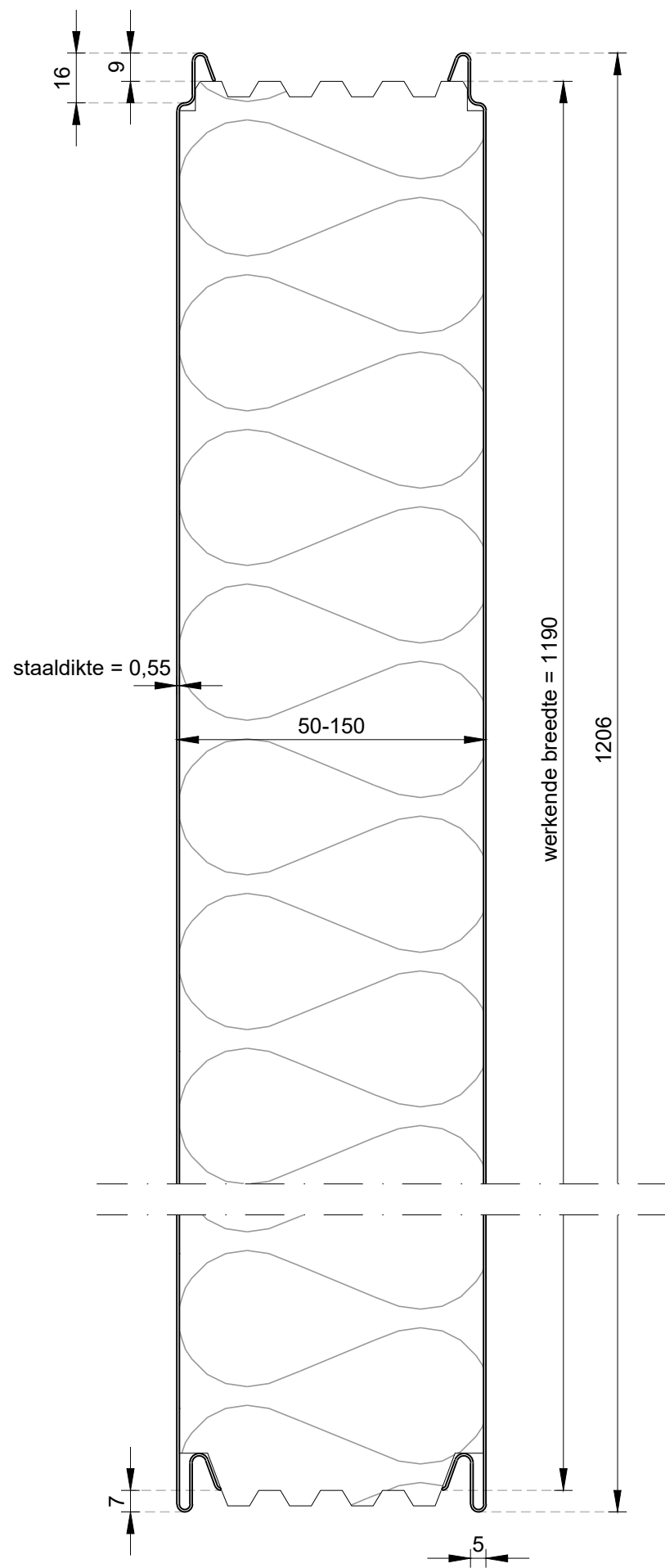
Doorsnede steenwol paneel
