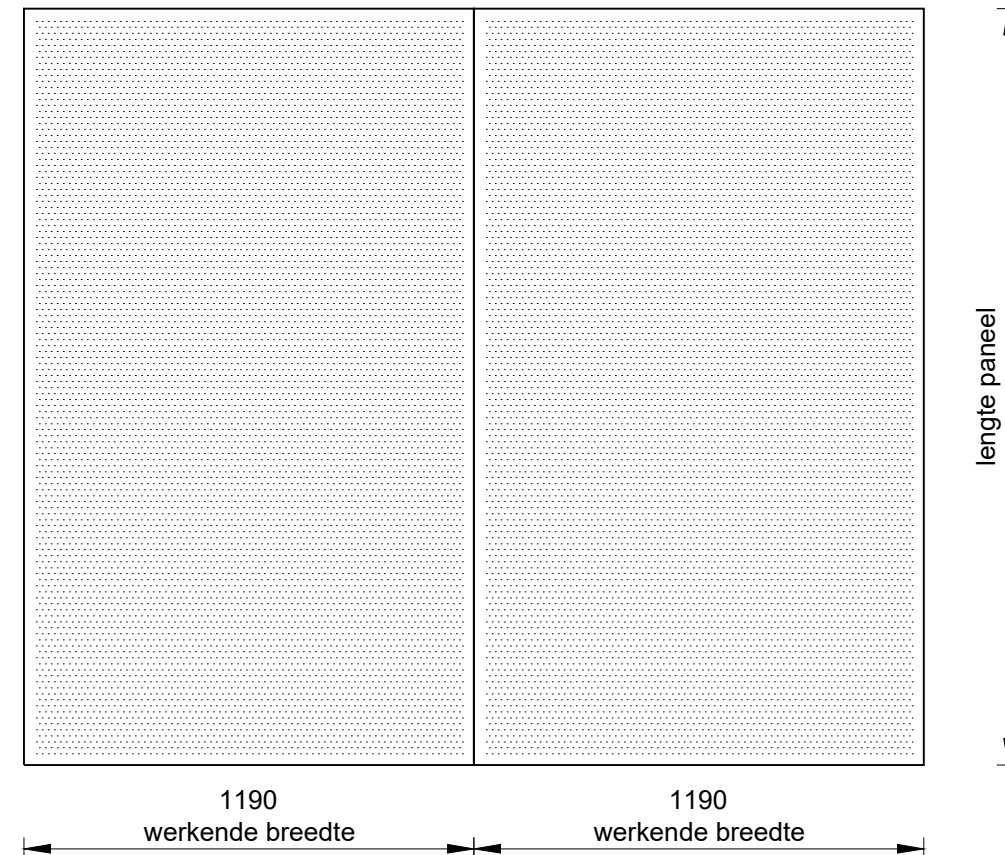
Aanzicht, eenzijdig geperforeerde steenwol paneel
