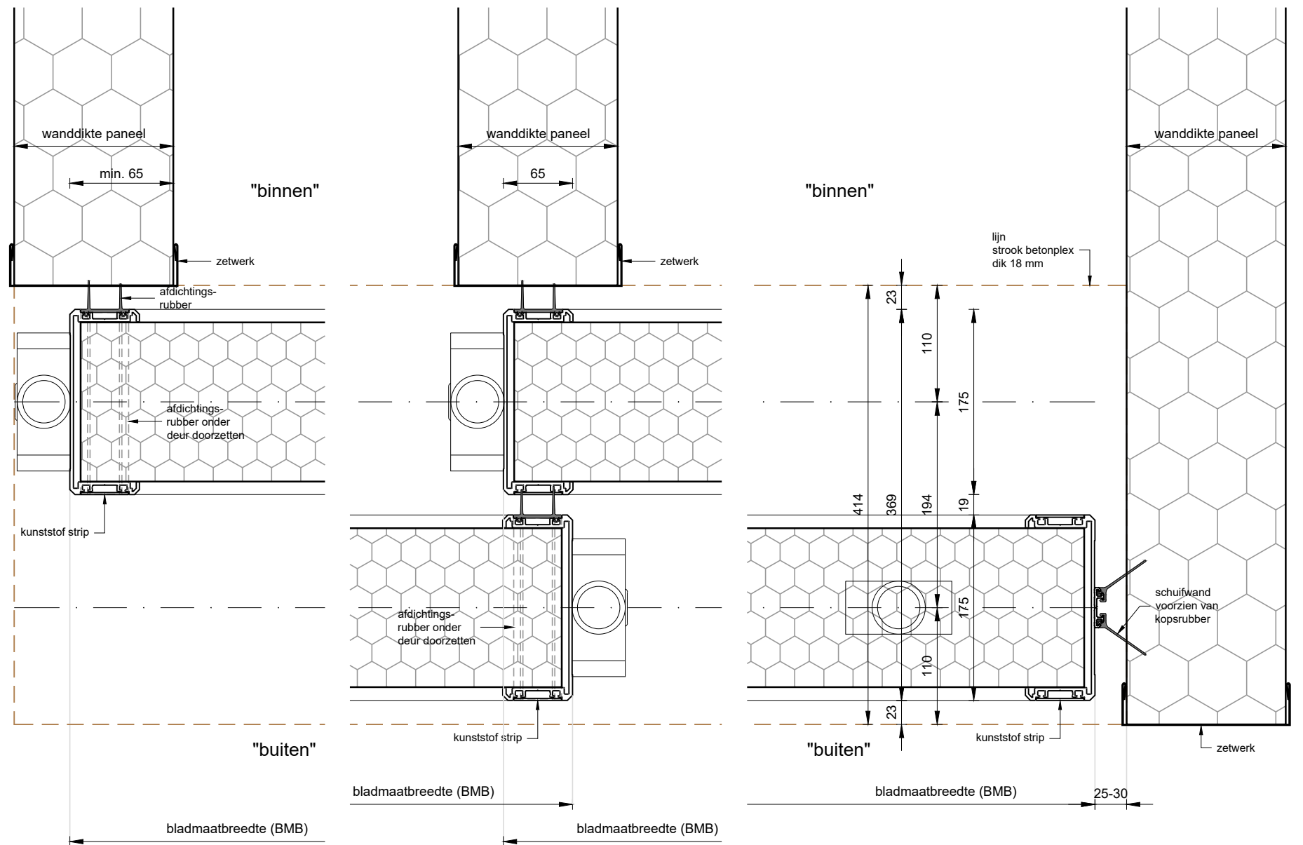
Principe details horizontaal schuifwand schaal 1:5
