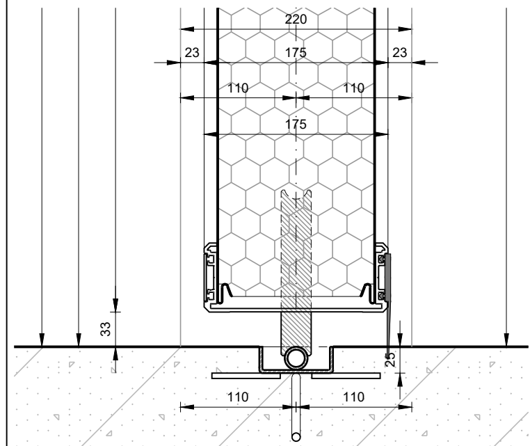
Principe details verticaal schuifwand, enkele rails schaal 1:5
