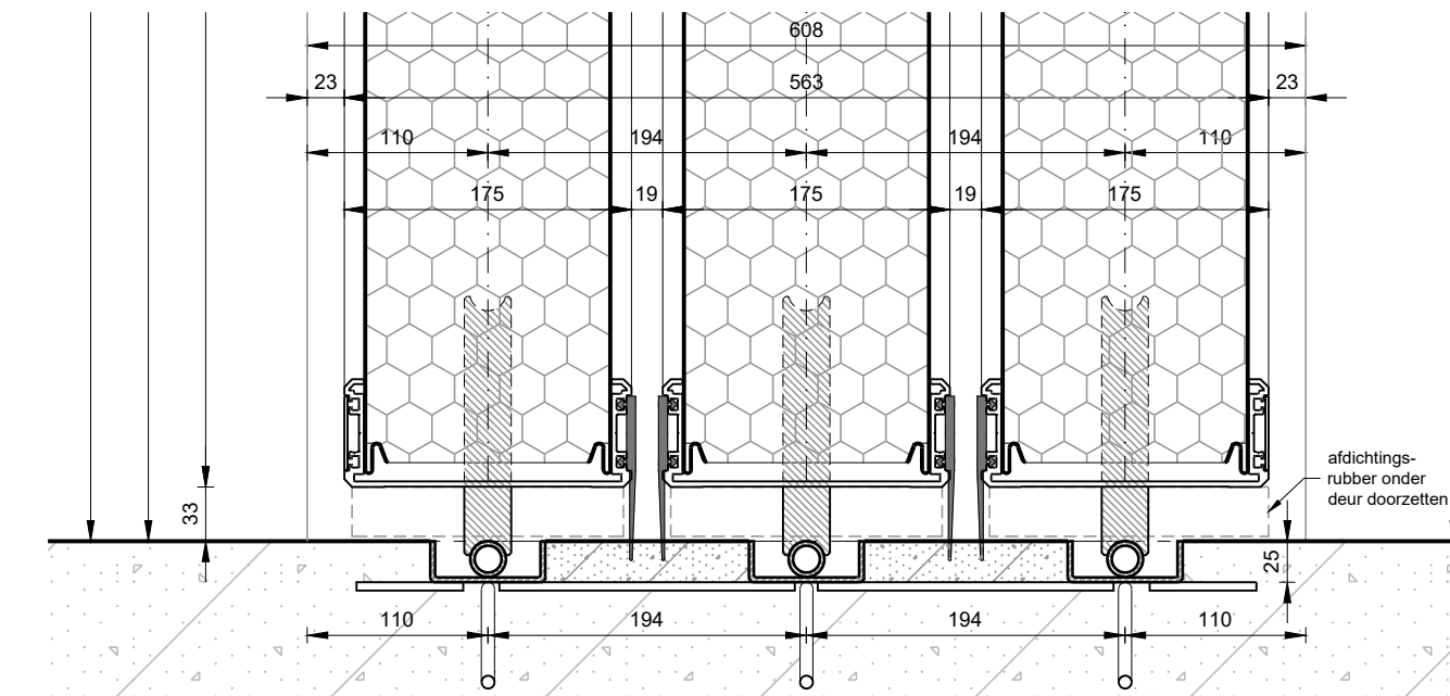
Principe details verticaal schuifwanden, triple rails schaal 1:5
