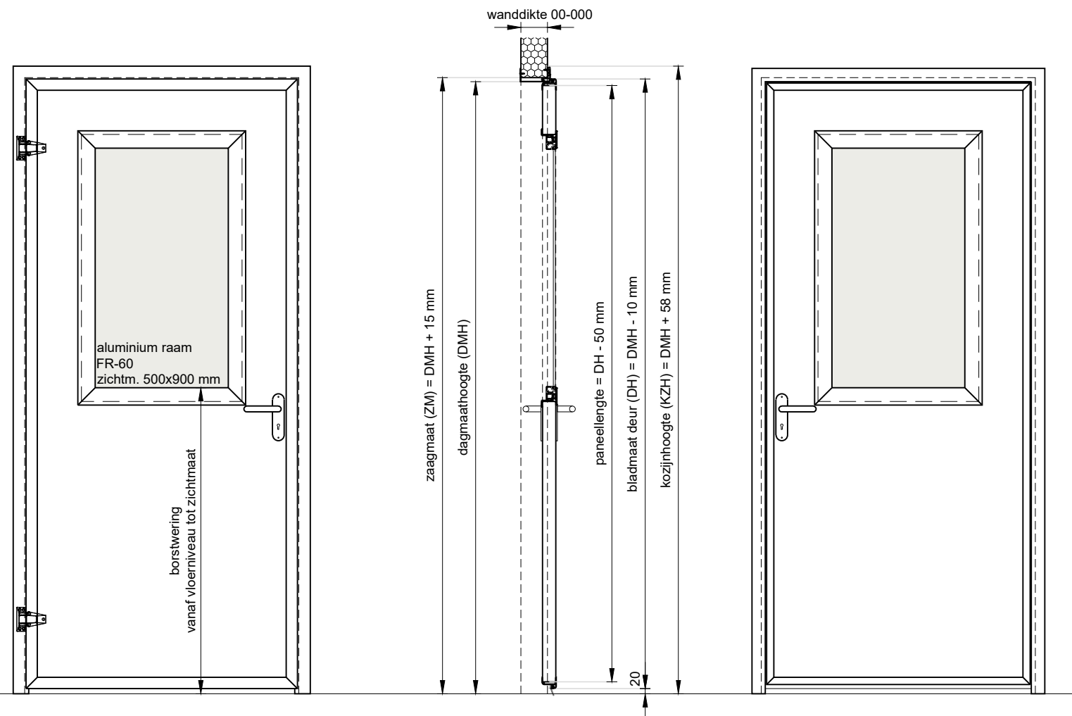
Vooraanzicht schaal 1:20
